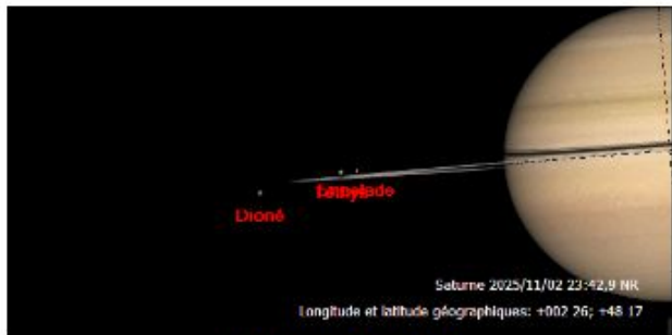
2 Novembre 2025 Encelade occulte Tethys ( 203 )
