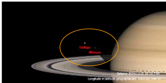
16 Novembre 2024 Mimas Eclipse Tethys ( 1E3 )
