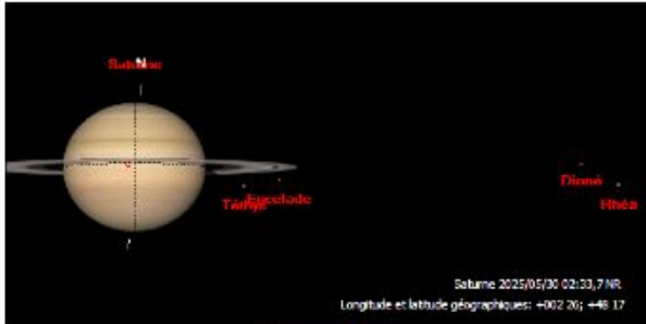
30 Mai 2025 Dione Eclipse Rhea( 4E5 )
