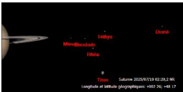
10 juillet 2025 Minas Eclipse Rhea( 1E5 )
