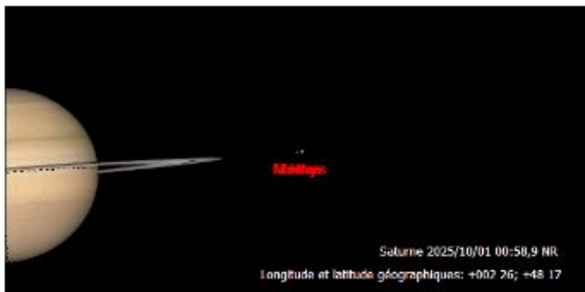
1 Octobre 2025 Tethys Occulte Minas ( 3O1 )
