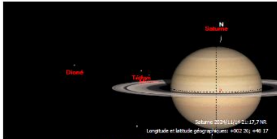
14 Novembre 2024 Mimas Eclipse Tethys ( 1E3 )
