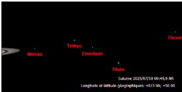
10 juillet 2025 Tethys Eclipse Encelade( 3E2 )
