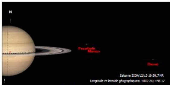
13 Decembre 2024 Mimas Eclipse Ecelade( 1E2 )
