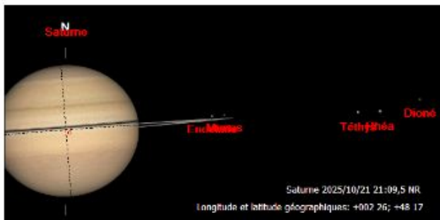
21 Octobre 2025 Encelade occulte Minas ( 201 ) Dans l'ombre ?
