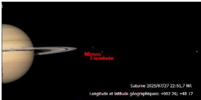
27 Juillet 2025 Minas Eclipse Encelade ( 1E2 )
