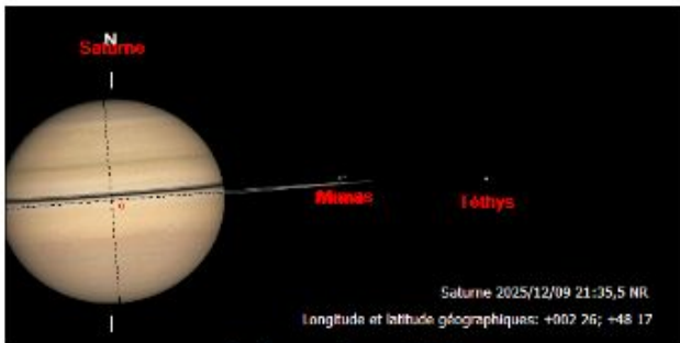
9 decembre 2025 Dione occulte Mimas ( 401 )
