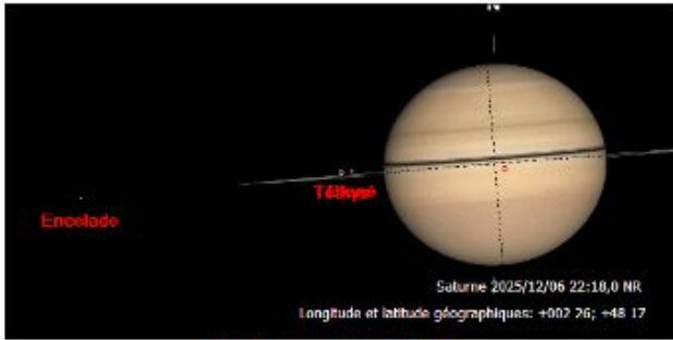
6 decembre 2025 Diane occulte Tethys ( 403 )
