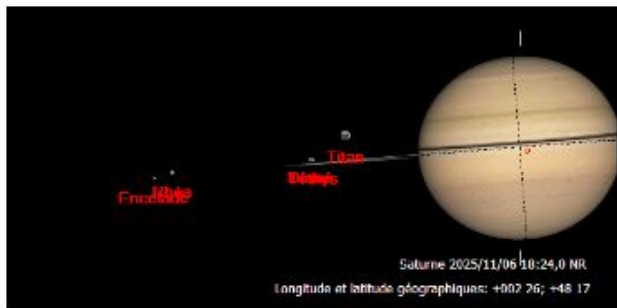
6 Novembre 2025 Diane occulte Tethys ( 403 )
