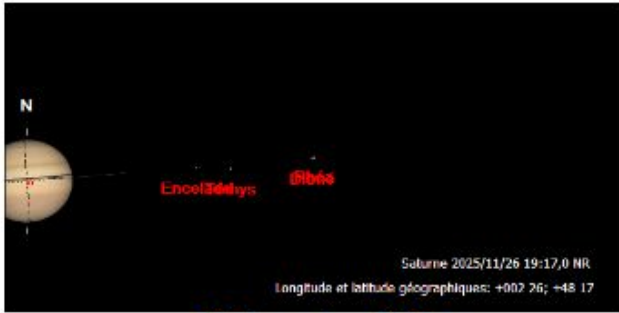
26 Novembre 2025 Dione Occulte Rhea( 405 )
